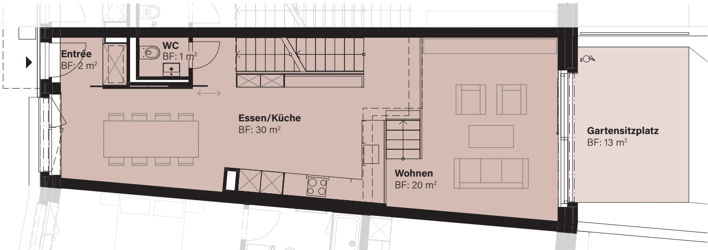
Erdgeschoss
