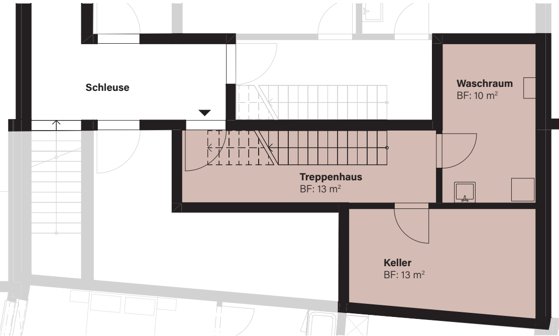
Untergeschoss
