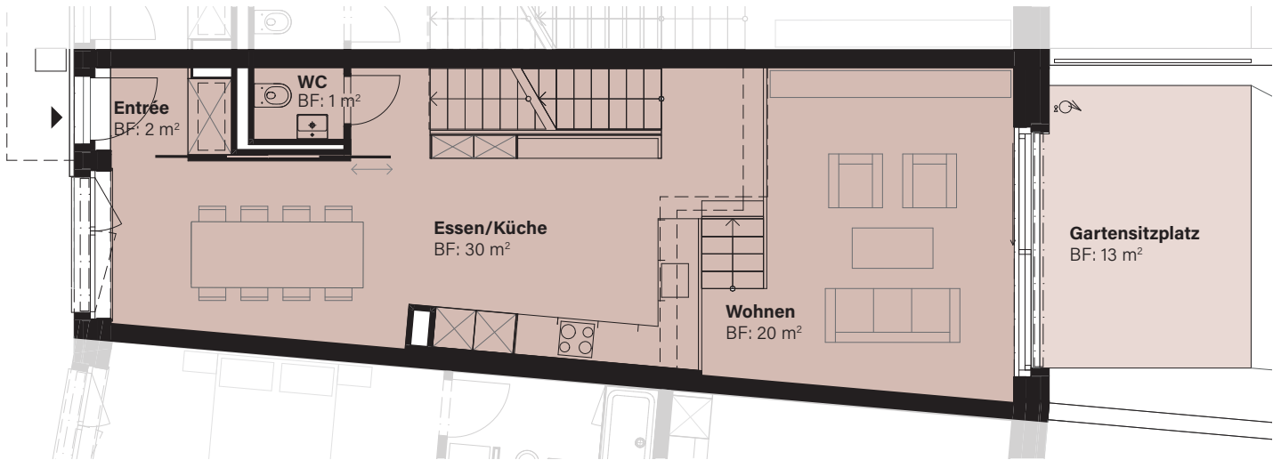
Erdgeschoss
