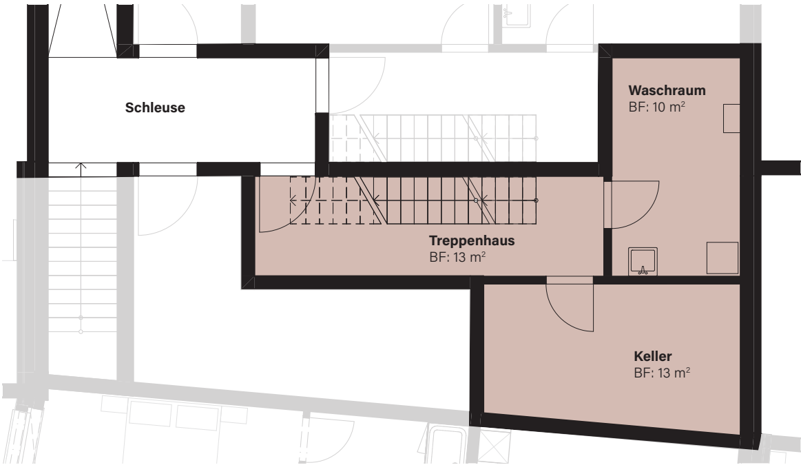
Untergeschoss
