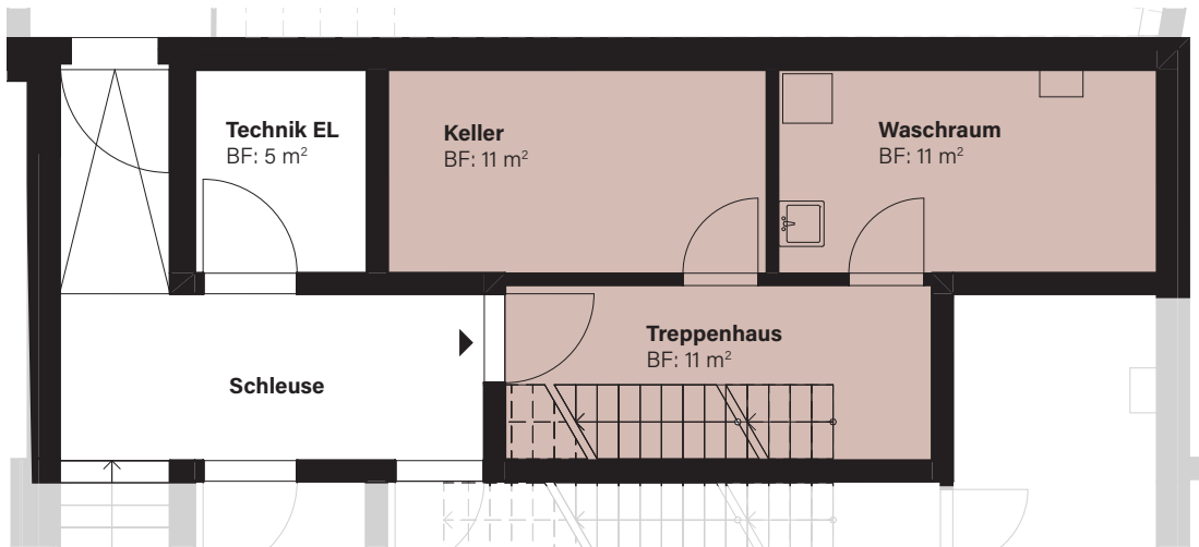
Untergeschoss
